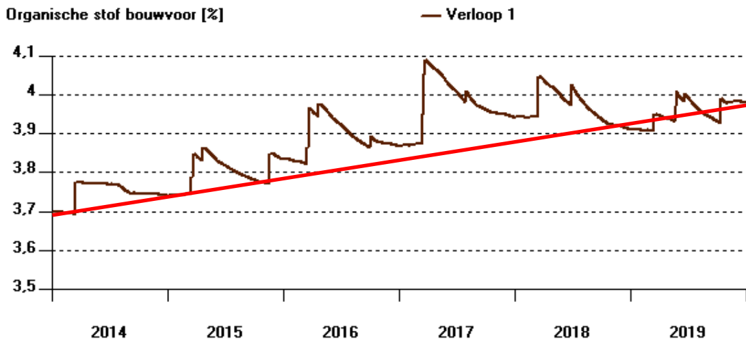
Figuur 13. Biologisch met compost, 1e rotatie. Verloop organische stof.
