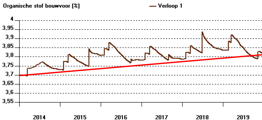
Figuur 3. Gl laag met compost, 1e rotatie. Verloop organische stof.
