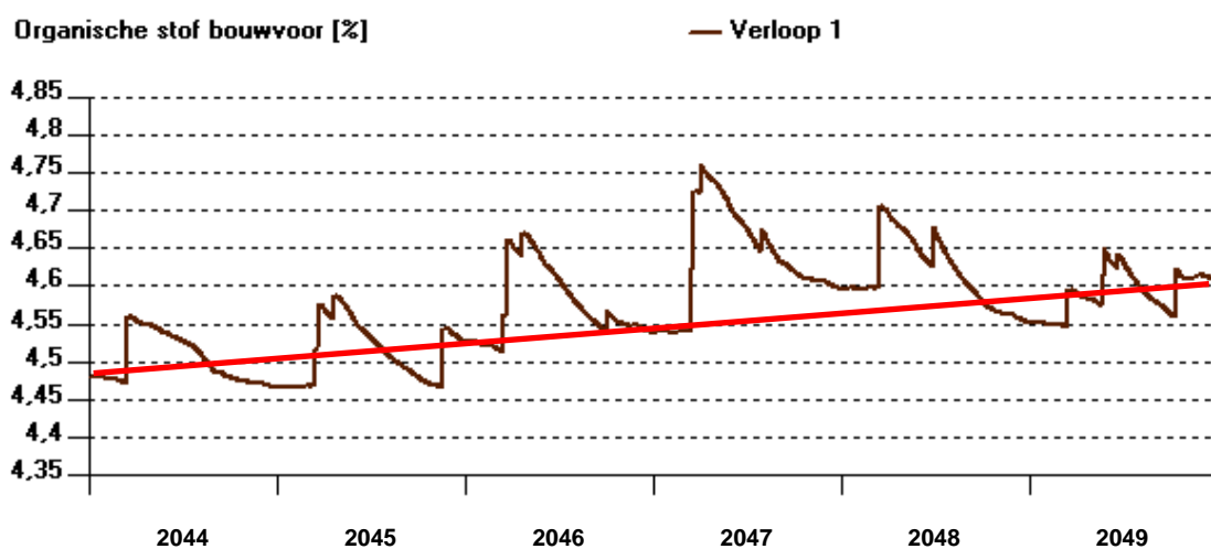
Figuur 15. Biologisch met compost, 6 e rotatie. Verloop organische stof.
