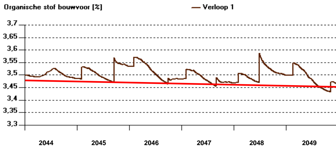
Figuur 4. GI laag zonder compost, 6e rotatie. Verloop organische stof.
